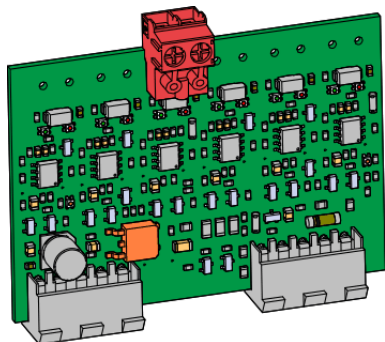
Abb./Fig. 1: TST SURA1 mit 5x 8,2 kΩ Abschlusswiderständen/TST SURA1 with 5x 8.2 kΩ terminating resistors/TST SURA1 avec 5x résistances terminales de 8,2 kΩ
